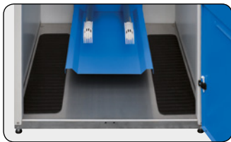
vyspádované nerezové podstava pre odvod vody a guma s priečnym dezénom proti podšmyknutiu
